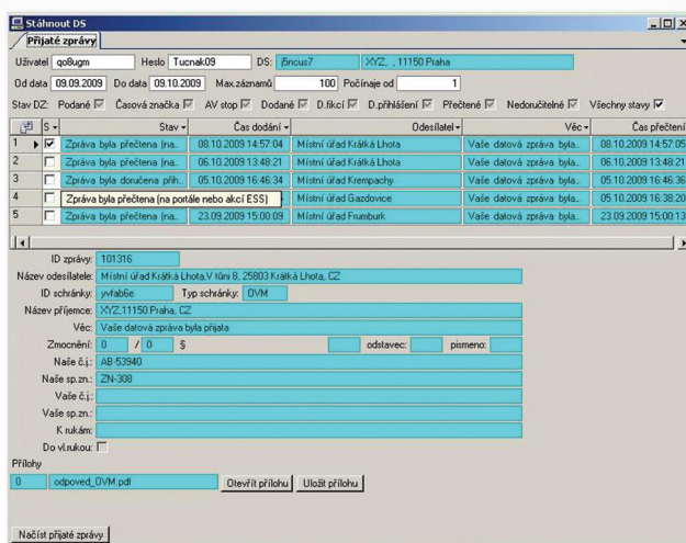
Obr 2. Funkce stažení zpráv z DS do Helios Green
