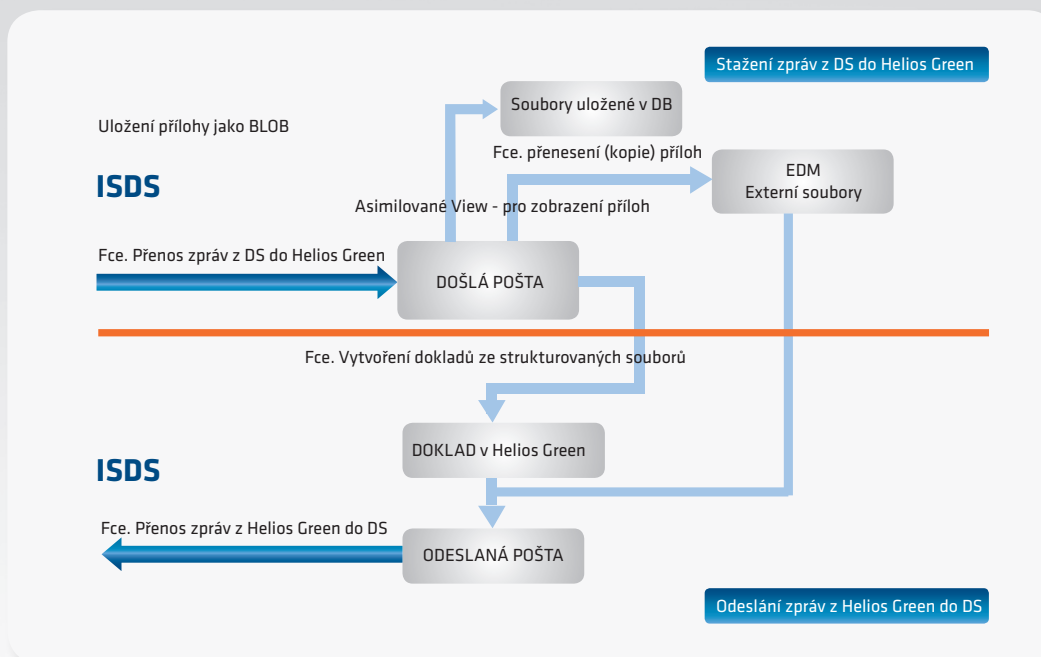
Obr 1. Schéma stažení a odeslání zpráv DS - Helios Green
